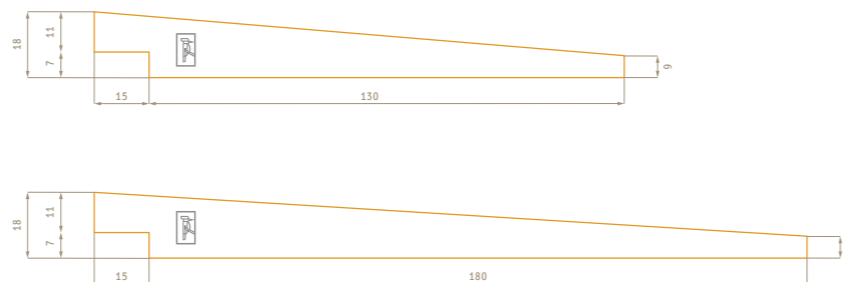
ZWEEDS RABAT
