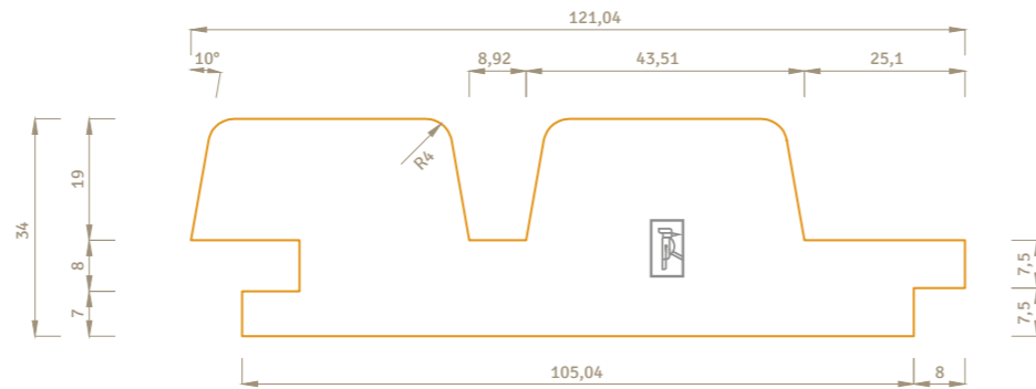
DUBBEL RHOMBUS
